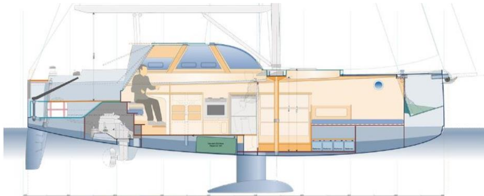
NOUVEAU MONDE 900 - AMENAGEMENTS Avant-Projet V3 Echelle : 1/25'
